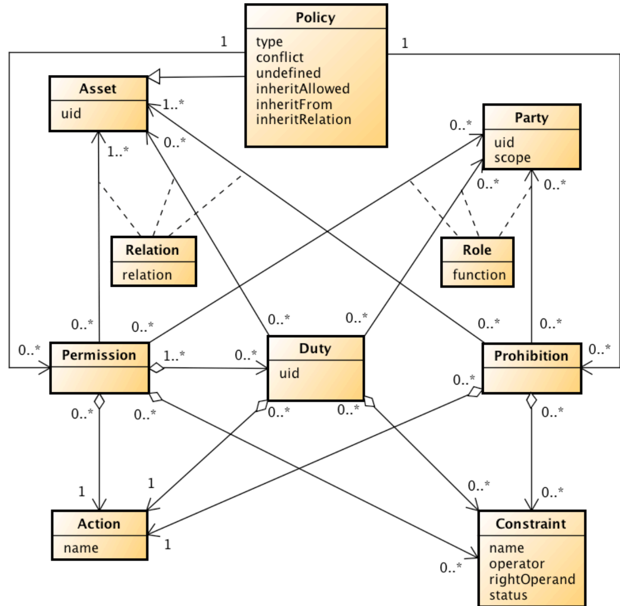
ODRL core model (W3C)
