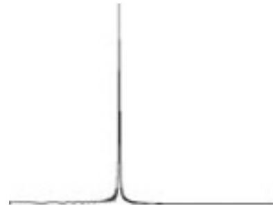
Sinus 110 Hz
